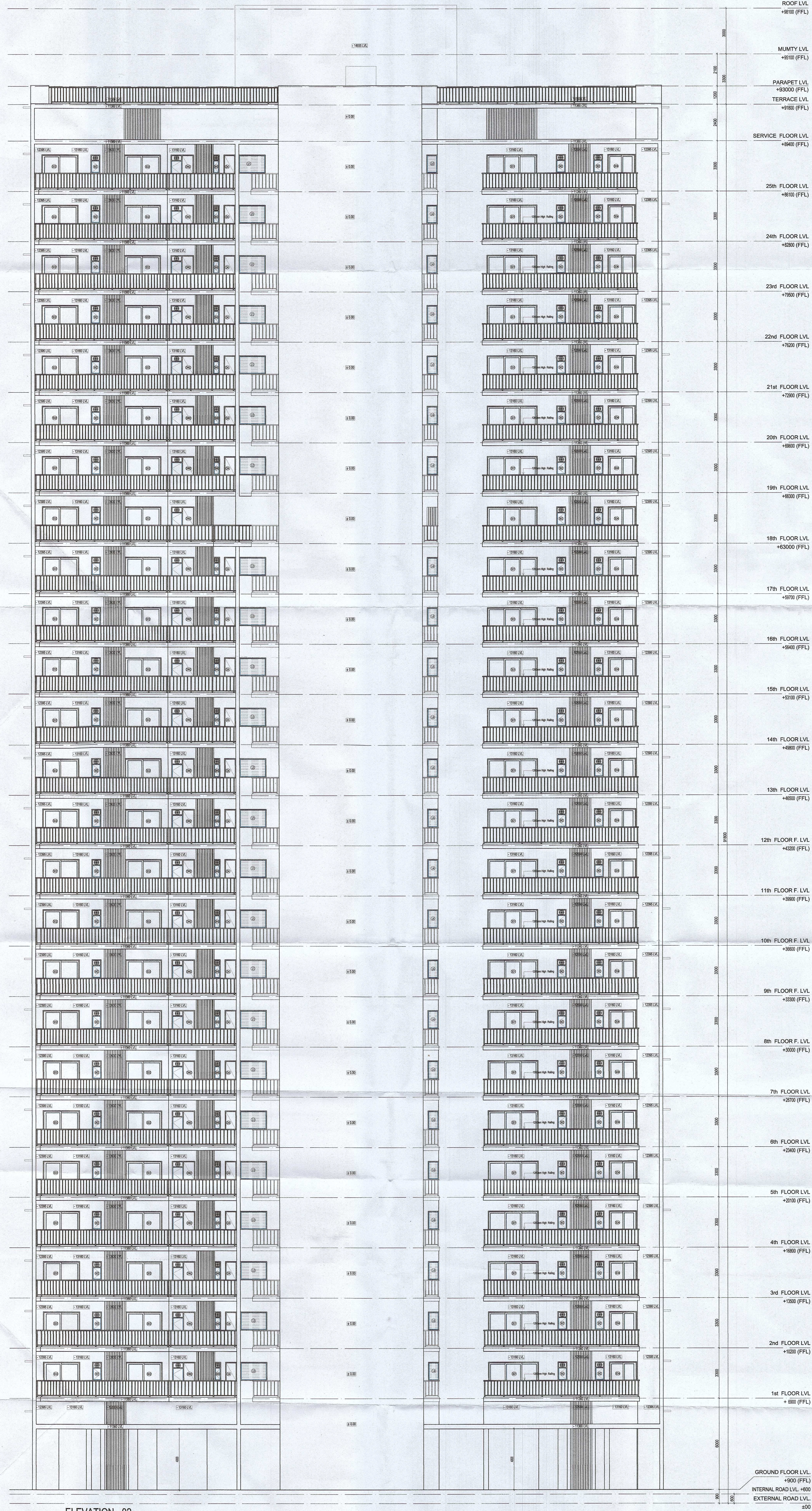
ELEVATION - 02
